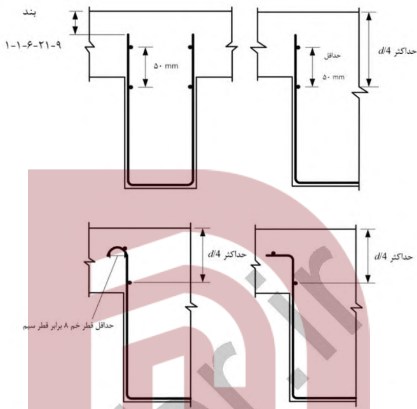
شکل ۱-۲۱-۹ مهار در ناحیه‌ی فشاری خاموت U شکل متشکل از شبکه‌ی سیمی ساده‌ی جوش شده
