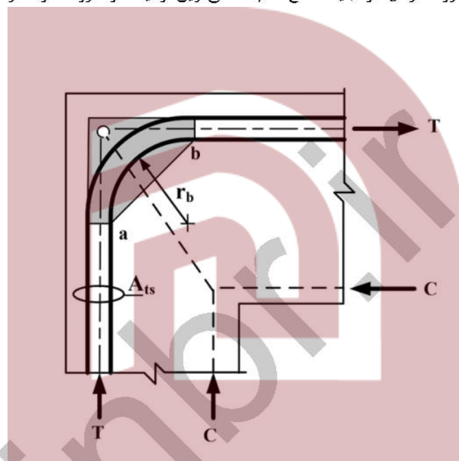
شکل ۹-۳-۹ شعاع داخلی خم برای چند ردیف میلگرد
