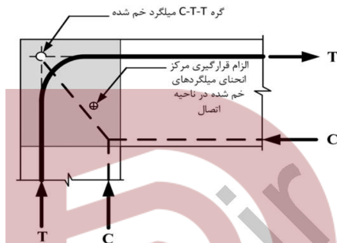
شکل ۹-۳-۱۰ الزام قرارگیری مرکز انحنای میلگردهای خم شده در ناحیه‌ی اتصال
