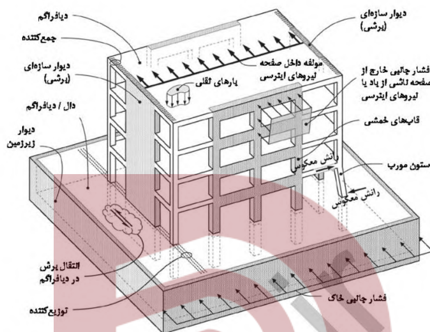
شکل ۱۴-۹ نیروهای وارد بر دیافراگم
