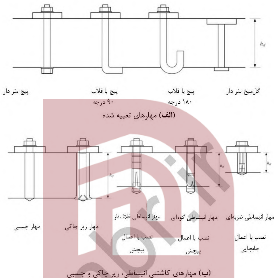
شکل ۹-۱۸-۱ انواع مهارها
