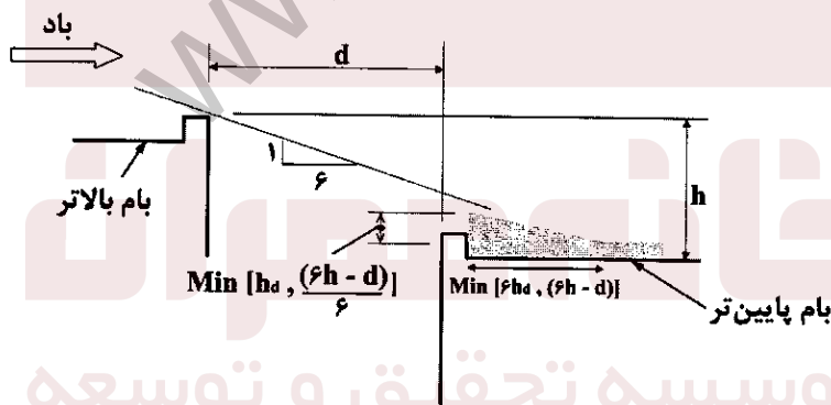
شکل ۶-۷-۹ بار انباشتگی برف پشت به باد روی بام پایین‌تر ساختمان مجاور
