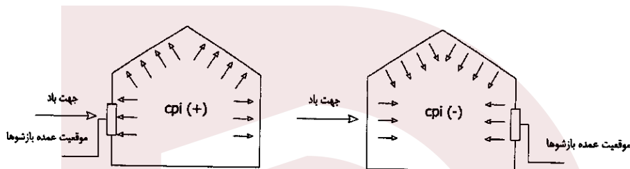
شکل ۶-۱۰-۱۲ ضریب اثر بارشو C_{pi}
