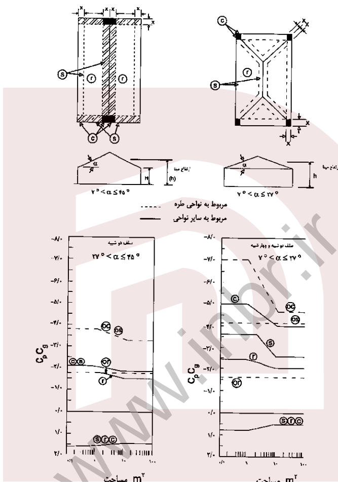
شکل ۶-۱۰-۷ ضرایب ترکیبی فشار و مکش خارجی C_p C_g برای طراحی پوشش‌ها و اجزاء بام (بام‌های دو شیبه یا چهار شیبه با زاویه شیب بیش از ۷ درجه)
