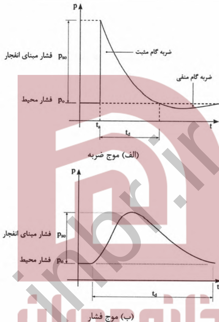
شکل ۲۱-۳-۱- شکل‌های موج ضربه و موج فشار
