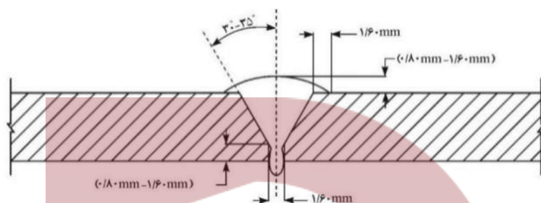
شکل ۱۷-۵-۱ طرح اتصال جوش لب به لب
