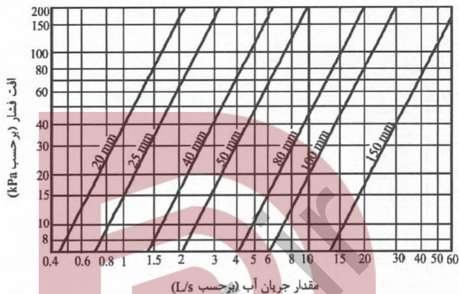
شکل پ ۱-۴-۲ (SI) - افت فشار در کنترلر نوع دیسکی بر حسب کیلوپاسکال
