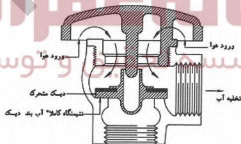
خلأشکن آتمسفریک در حالت مکش سیفونی
