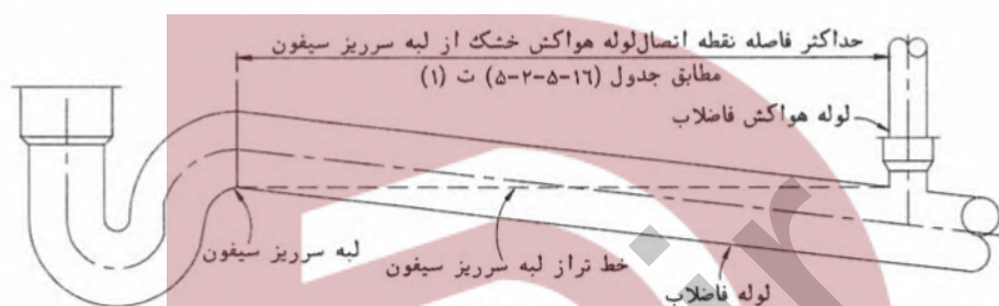
شکل ۵-۲-۵-۱۶ "ت" - اتصال لوله هواکش خشک لوازم بهداشتی
