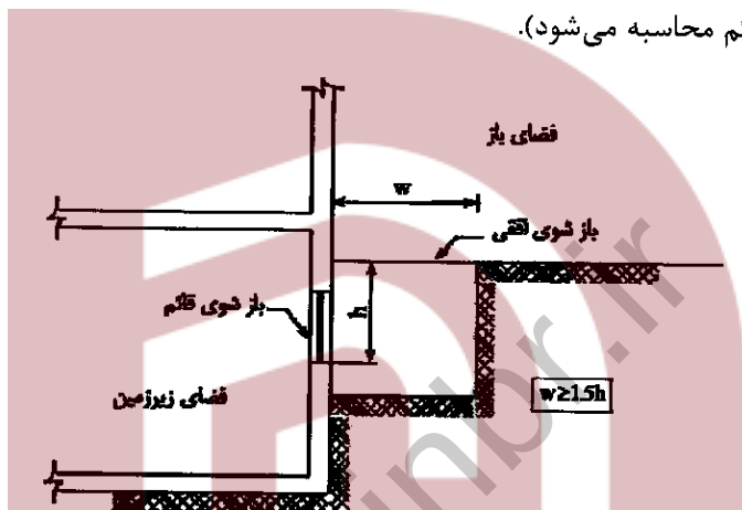
شکل (۳-۳-۴-۱۴): تعویض هوای طبیعی فضای واقع در زیرزمین
