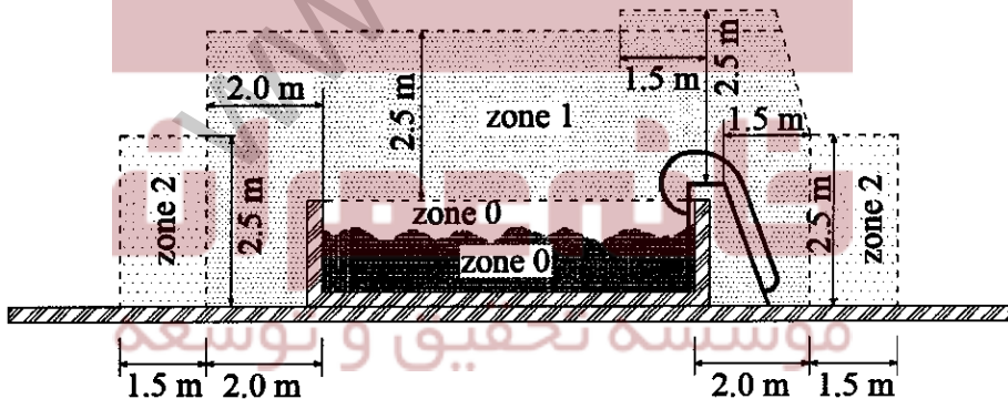
شکل ۱۰-۱۳-۶: طرحواره ابعاد مناطق (zone) برای استخر احداث شده روی کف زمین (دید از کنار)
