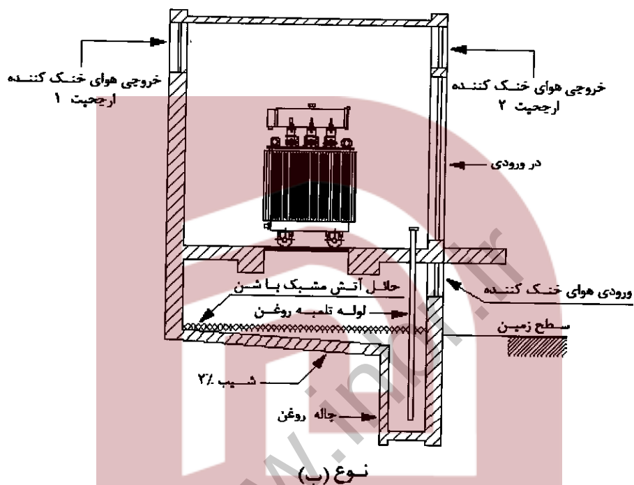
شکل ۱۳-۵-۳: (نوع ب) - طرحواره مقطع قائم اتاق ترانسفورماتور روغنی با تهویه مکانیکی و بالاتر از سطح زمین
