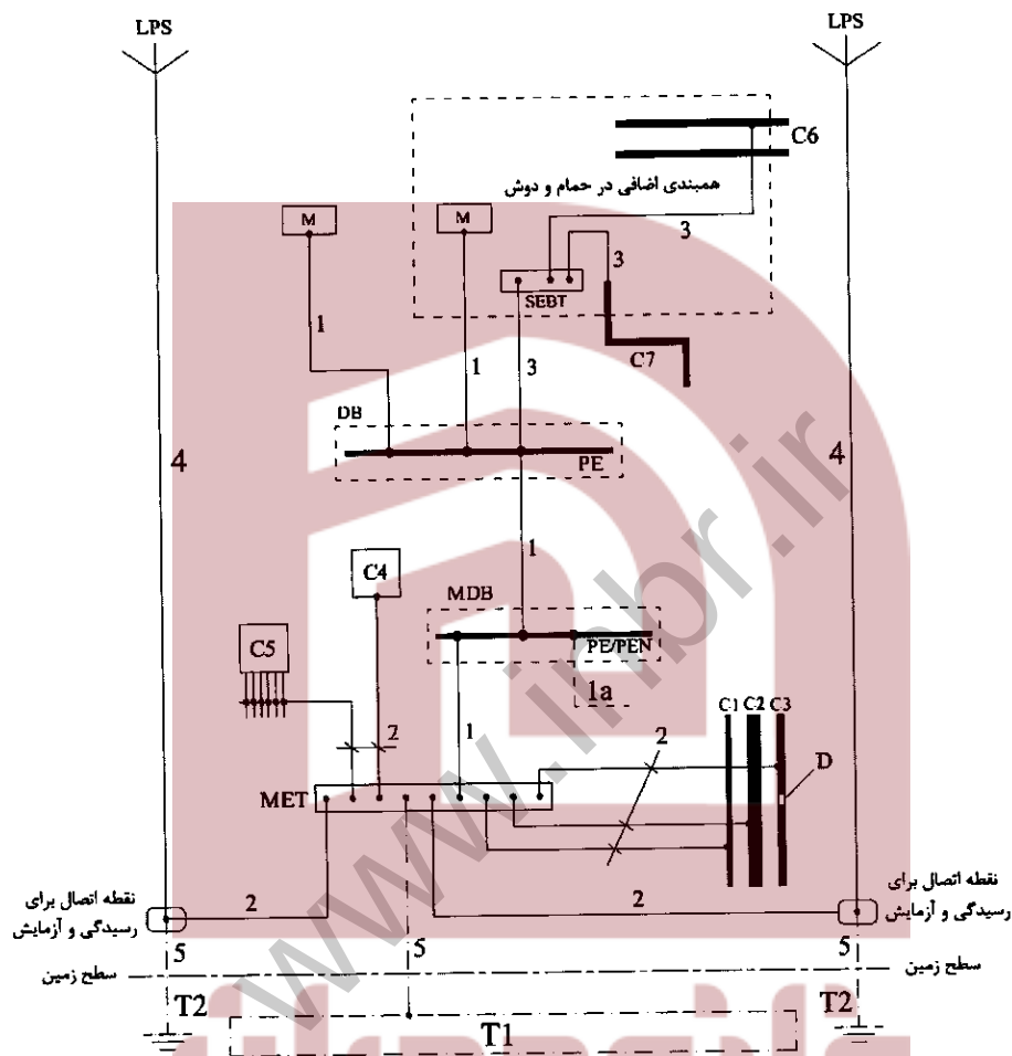
شکل پ ۱-۲-۴ طرحواره عمومی هم‌بندی اصلی و اضافی برای هم‌ولتاژ کردن موسسه تحقیق و توسعه
