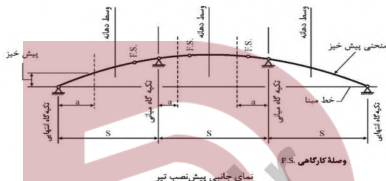
شکل ۱۰-۴-۱۱: روش اندازه‌گیری پیش‌خیز تیرها
