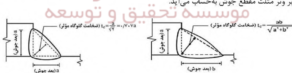
شکل ۱۰-۹-۲-۹: بعد و ضخامت گلوگاه مؤثر جوش‌های گوشه
