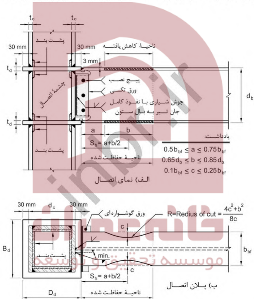
شکل ۱۰-۷-۳-۱: اتصال گیردار تیر با مقطع کاهش یافته و دیافراگم عبوری از ستون (TD-RBS)
