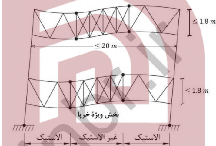
شکل ۱۰-۳-۳-۴: سازوکار تسلیم در بخش ویژه خرابا و رفتار ارتجاعی در سایر بخش‌های خرابا و ستون قاب
