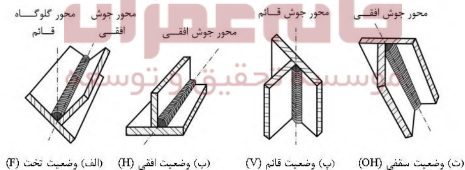
شکل ۱۰-۴: چهار وضعیت اصلی جوشکاری برای جوشکاری با جوش گوشه
