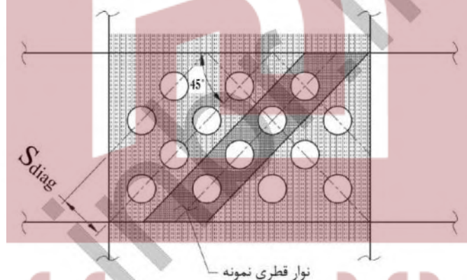
شکل ۱۰-۳-۴-۵: آرایش سوراخ‌ها در دیوارهای برشی فولادی ویژه سوراخ‌دار
