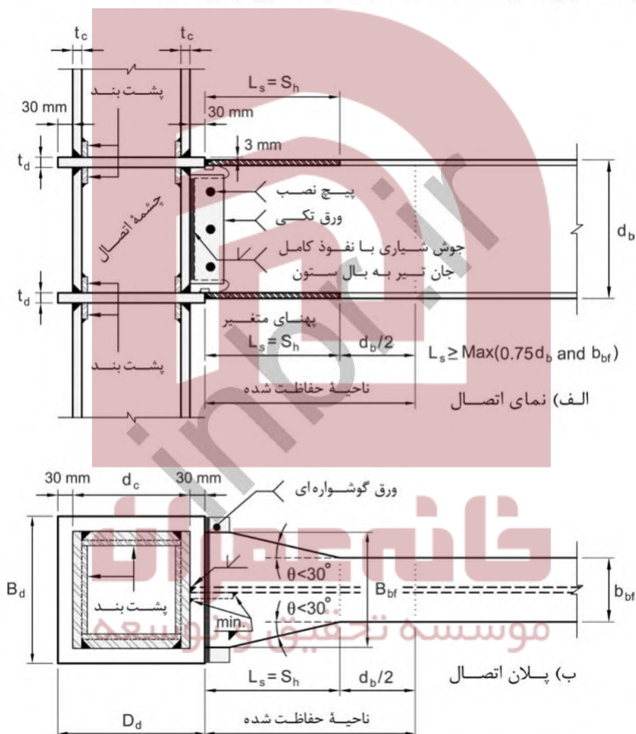
شکل ۱۴-۷-۳-۱۰: اتصال گیردار تیر با بال پهن شده و دیافراگم عبوری از ستون (TD-WIDENED)
