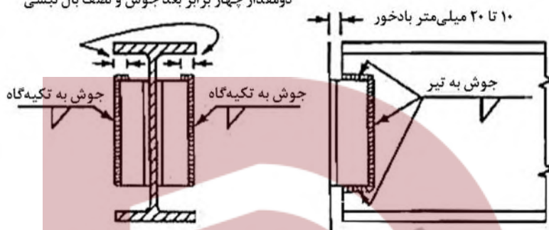
شکل ۱۰-۲-۵: جزئیات اتصال جوشی با استفاده از نبشی جفت در جان
