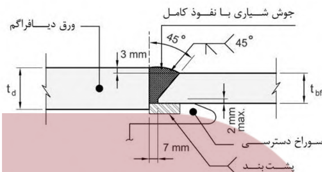
شکل ۱۰-۳-۷-۱۱: اتصال بال تیر به ورق دیافراگم با استفاده از سورخ دسترسی و ورق‌های پشت‌بند
