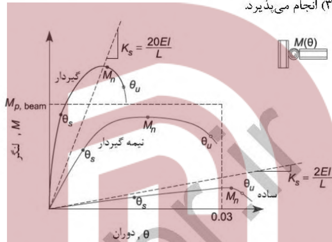
شکل ۲-۱۰-۳-۹: نمونه منحنی لنگر-دوران و دسته‌بندی اتصالات
