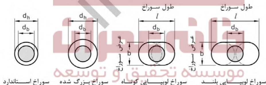
شکل ۱۰-۲-۹-۱۵: انواع سوراخ پیچ‌ها در اتصالات پیچی
