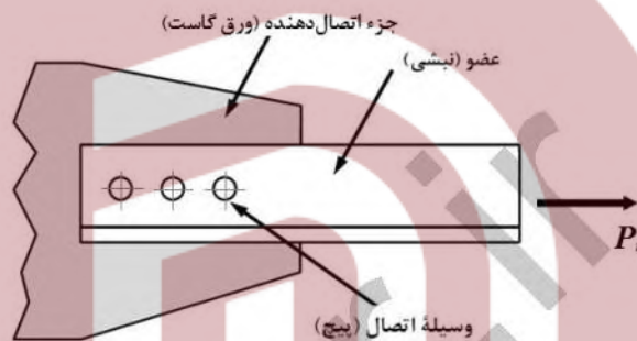
شکل ۱۰-۲-۹-۱: نام‌گذاری قسمت‌های مختلف یک اتصال
