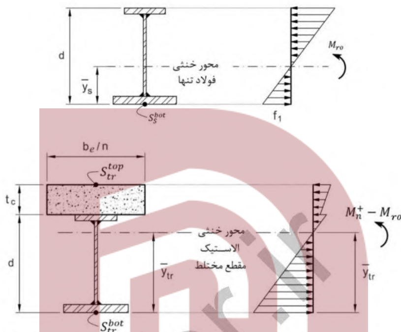
شکل ۵-۲-۱۰ توزیع الاستیک تنش در مقطع مختلط تبدیل یافته در صورت عدم استفاده از پایه‌های موقت
