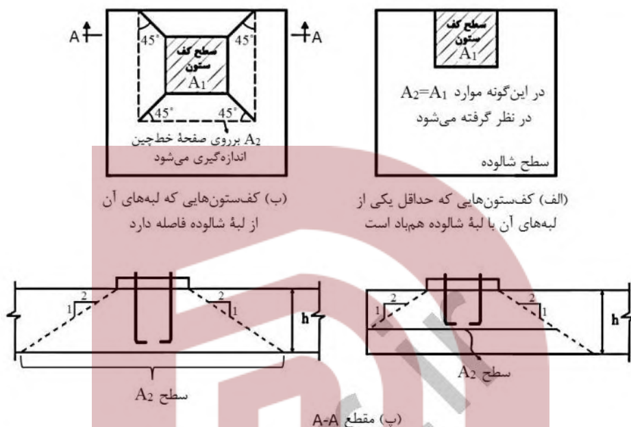
شکل ۲-۱۰-۹-۲۲: سطح اتکا در تماس با تکیه‌گاه بتنی
