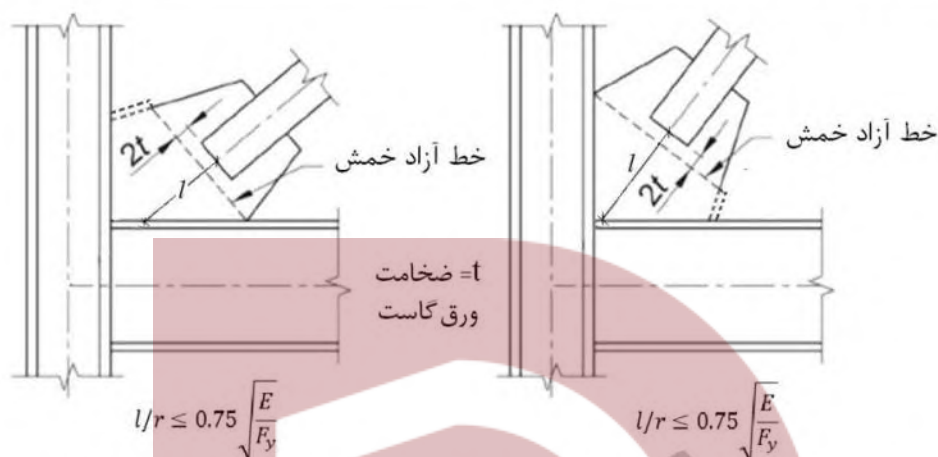
شکل ۳-۱۰-۳-۴-۲: سازگاری ورق اتصال (ورق گاست) با کمانش خارج از صفحه عضو مهاربندی
