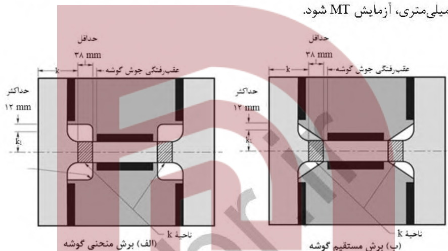
شکل ۱۰-۴-۲۶: جوشکاری خارج ناحیه K در محل اتصال ورق پیوستگی
