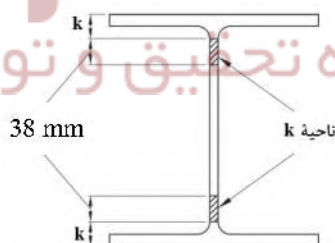
شکل ۴-۱۰: ناحیه k
