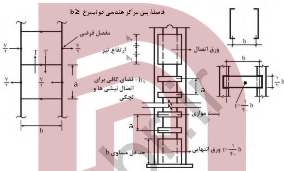
شکل ۱۰-۲-۴-۴: عضو فشاری ساخته‌شده (مرکب) با بست‌های موازی
