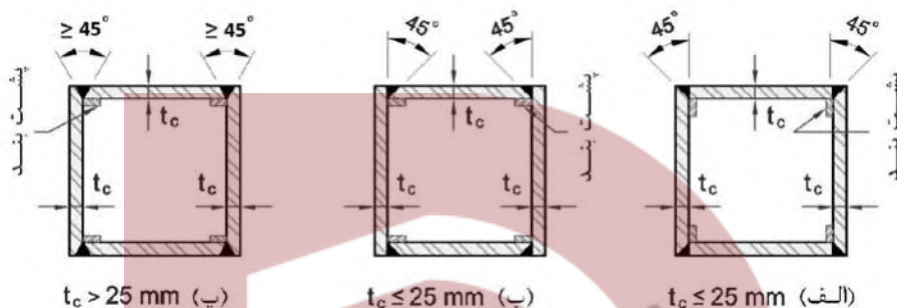
شکل ۱۰-۷-۳: نحوه ساخت ستون‌های جعبه‌ای ساخته شده از ورق
