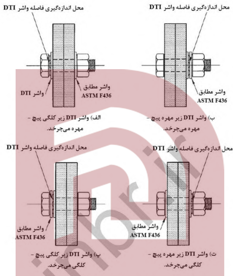
شکل ۱۰-۴-۶: محل قرار گرفتن واشر در روش DTI
