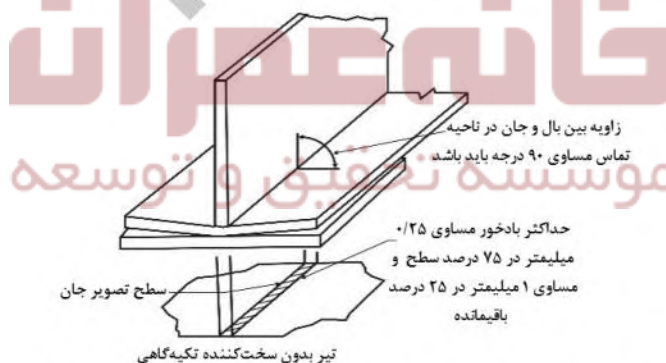
شکل ۴-۱۰-۱۵: رواداری در محل تماس تیر با تکیه‌گاه - تیر بدون سخت‌کننده تکیه‌گاهی
