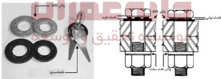
شکل ۱۰-۴-۷: فاصله قابل مشاهده در روش DTI پس از پیش تنیده کردن
