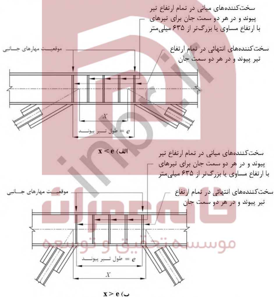
شکل ۳-۱۰-۳-۴-۳: تیر پیوند با مقطع I شکل و سخت‌کننده‌های موردنیاز
