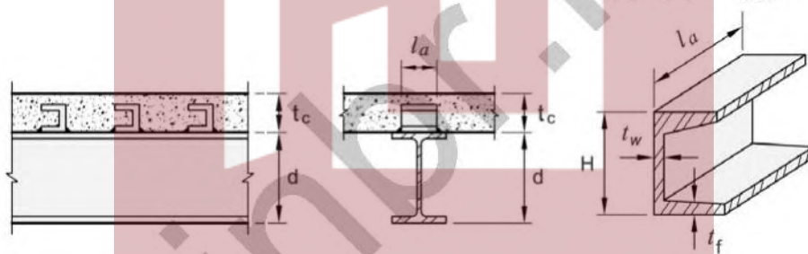
شکل ۱۰-۲-۸: برشگیرهای از نوع ناودانی
