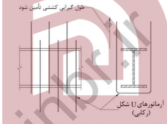
شکل ۳-۳-۶-۳-۱۰: استفاده از آرماتورهای U شکل به عنوان میلگردهای انتقال
