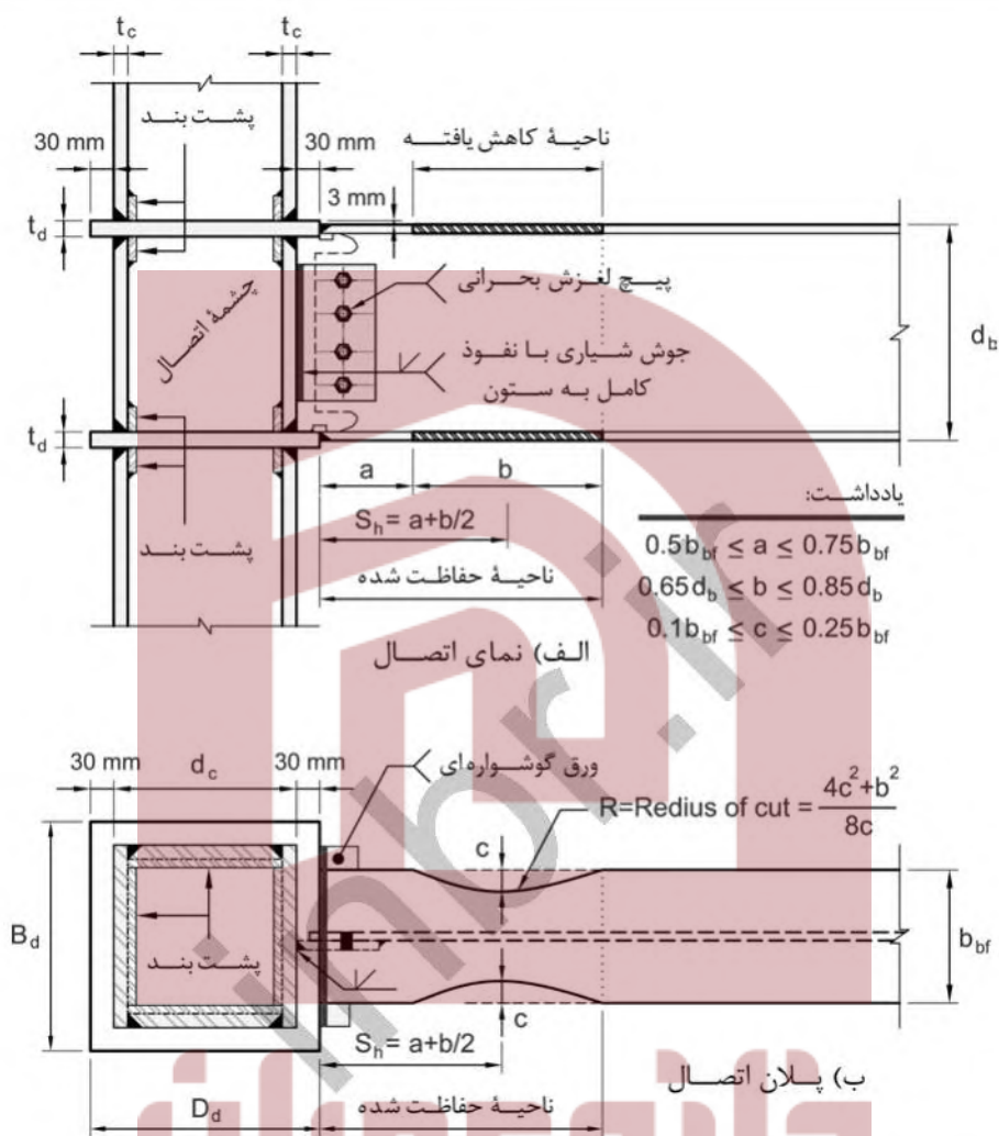
شکل ۱۰-۳-۷: اتصال گیردار تیر با مقطع کاهش یافته و دیافراگم عبوری از ستون در قاب‌های خمشی
